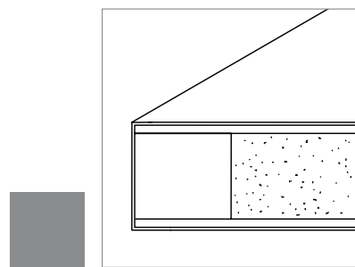
TRENDLINE flach geschnitten, ohne Falz
