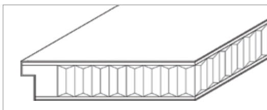
Türblatt mit Wabe als Mittellage
