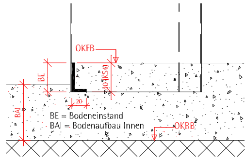
Konterschwelle (Typ I) --> alle Zargentypen
