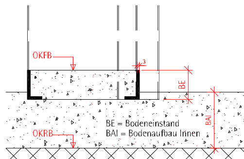
Doppelschwelle dichtungsbündig im 1. Falz "Doppelfalz" (Typ N) --> UD + UDS Zarge
