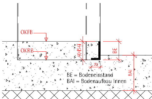
Schwelle spiegelbündig (Typ C) --> alle Zargentypen
