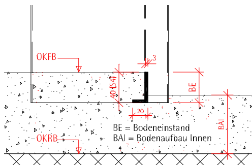
Schwelle dichtungsbündig (Typ F) --> UD + UDS Zarge
