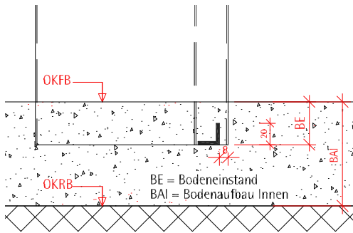
Schwellenlos prov. Verbindung geschweisst (Typ A) --> alle Zargentypen
