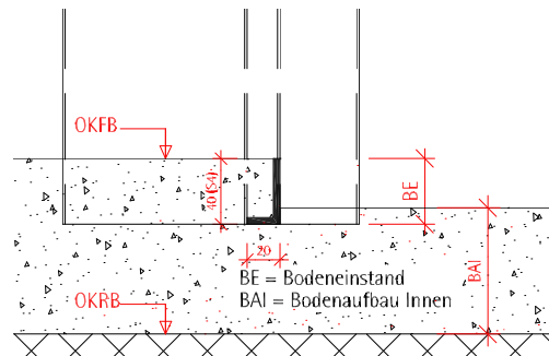
Schwelle nach Zafagnorm (Typ H4) --> UDDS Zarge
