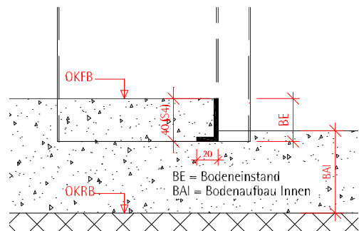
Schwelle falzbündig (Typ D) --> UD + UDS Zarge
