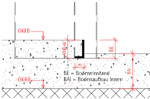
Schwelle nach Zafagnorm (Typ H3) --> UDS Zarge
