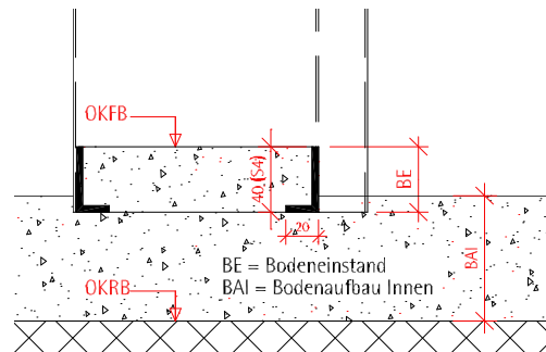
Doppelschwelle falzbündig (Typ K) --> UD + UDS Zarge
