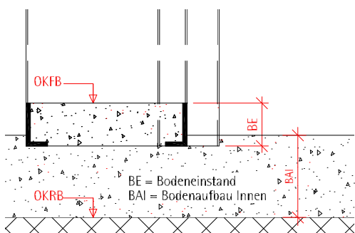
Doppelschwelle falzbündig im 1. Falz "Doppelfalz" (Typ L) --> UDD + UDDS Zarge
