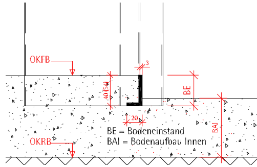
Schwelle dichtungsbündig im 1. Falz (Typ G) --> UD + UDS Zarge
