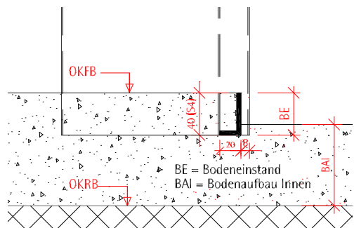
Schwelle nach Zafagnorm (Typ H1) --> UD Zarge
