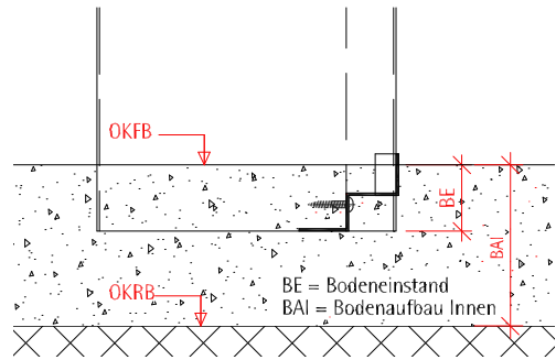
Schwellenlos prov. Verbindung geschraubt (Typ B) --> alle Zargentypen
