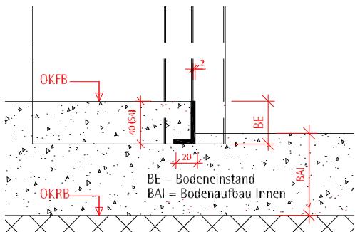
Schwelle nach Zafagnorm (Typ H2) --> UDD Zarge
