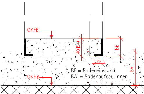
Doppelschwelle spiegelbündig (Typ J) --> alle Zargentypen
