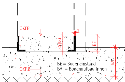
Doppelschwelle dichtungsbündig (Typ M) --> UD + UDS Zarge
