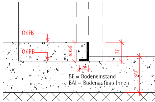
Schwelle falzbündig im 1. Falz (Typ E) --> UDD, UDDS Zarge
